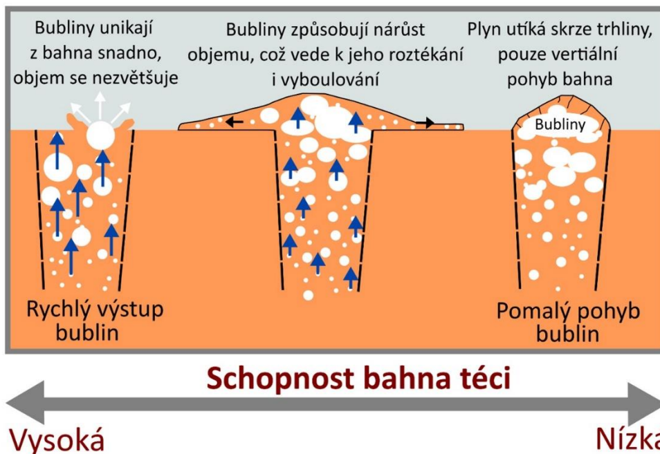
Bahna, které mají v sobě málo vody a jsou tedy velice hustá, v podstatě nedovolují vznikajícím bublinám vodní páry. Proto se jejich objem po vystavení sníženému atmosférickému tlaku dramaticky zvětší. Výsledkem může být útvar, který na první pohled sice vypadá jako sušenka, ale ve skutečnosti jde o bahnitý blob ze zmrzlé krusty a s kapalným nitrem plným velkých bublin. FOTO: Petr Brož
