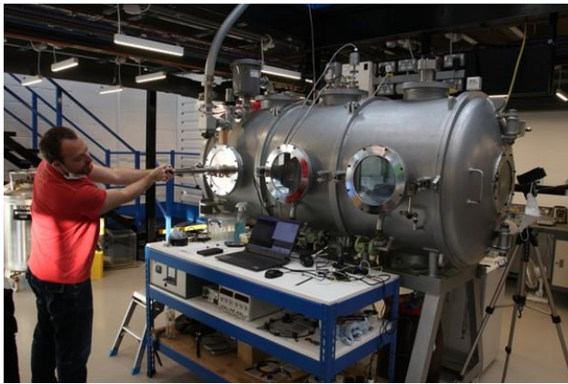
Pohled na nízkotlakovou komoru v britské Open University, ve které se pokusy s bahnem dělaly. Na snímku je jeden ze spoluautorů – Ondřej Krýza z Geofyzikálního ústavu AV ČR. Komora umožňuje snížit atmosférický tlak na průměrné hodnoty panující na povrchu Marsu během pár minut. FOTO: Petr Brož
